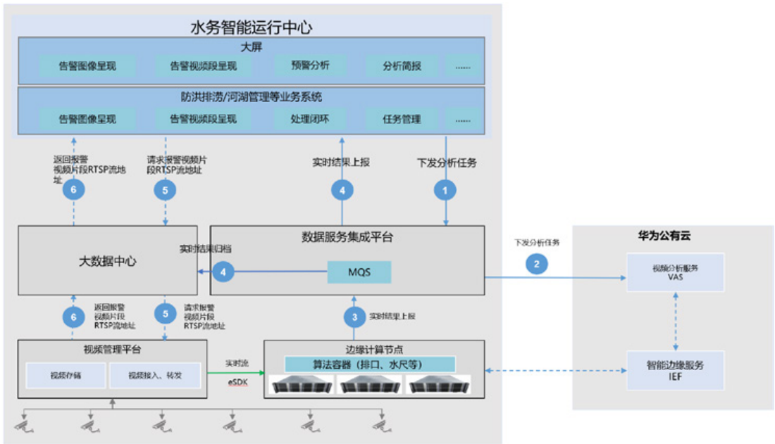
图 13-14 水务视频 AI 解决方案架构
