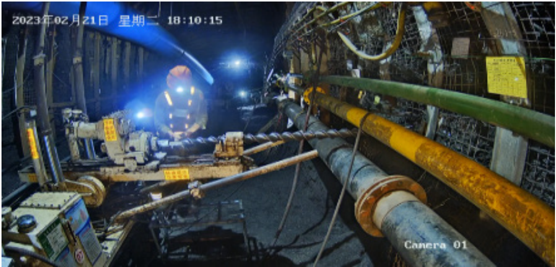
图 6-5 防冲卸压施工现场
