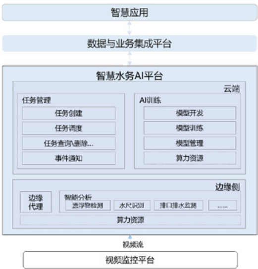
图 4-16 智慧水务 AI 解决方案架构图
