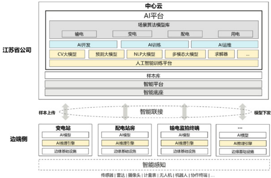
图 8-2 国网江苏省电力人工智能平台云边协同架构
