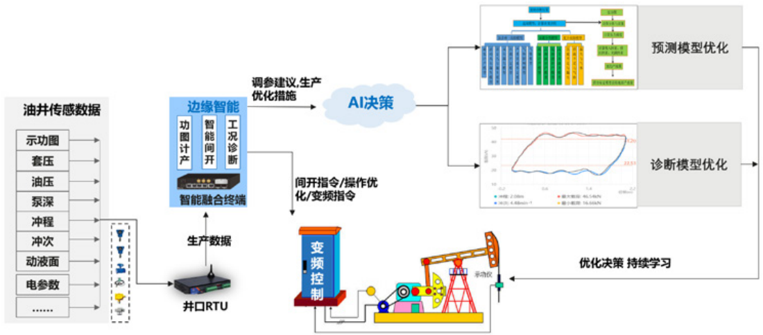
图 9-5 抽油机工况诊断业务流程
