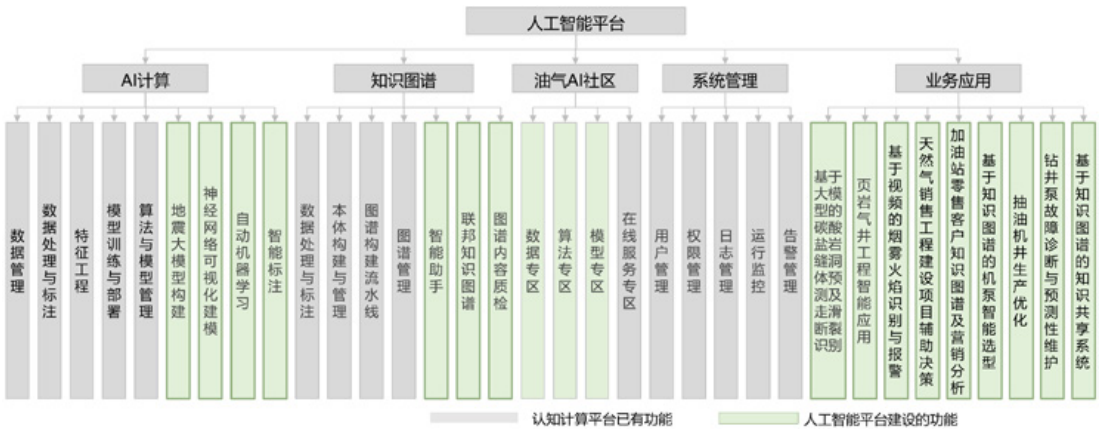
图 9-2 中国石油集团人工智能平台功能规划
