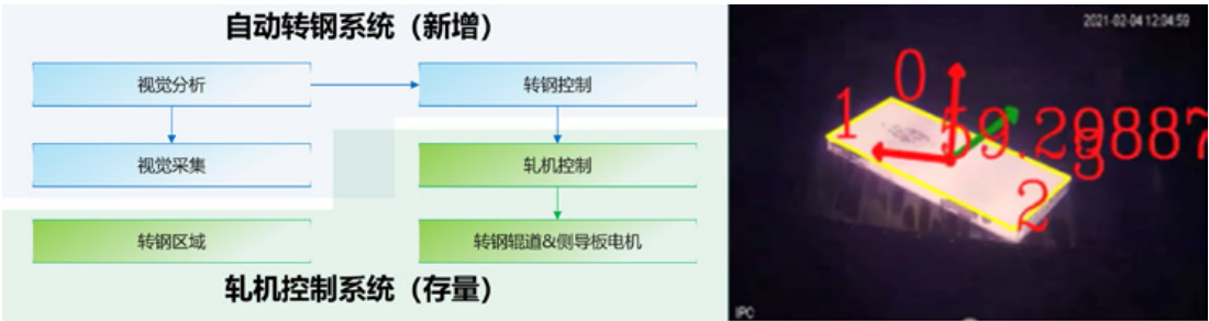
图 6-14 自动转钢原理（左图）& 实时纪录角度计算（右图）
