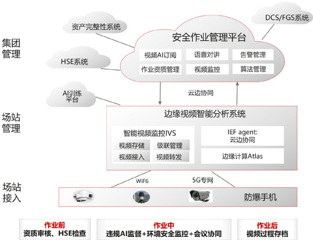
图 9-8 作业风险识别算法云边协同架构
