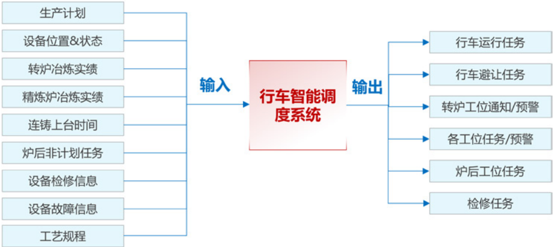
图 6-12 行车智能调度系统功能
