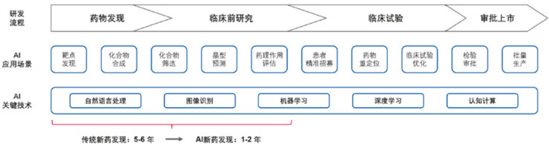
图 4-12 药物研发流程
