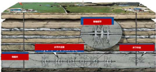
图 3-19 油气井射孔压裂剖面示意图
