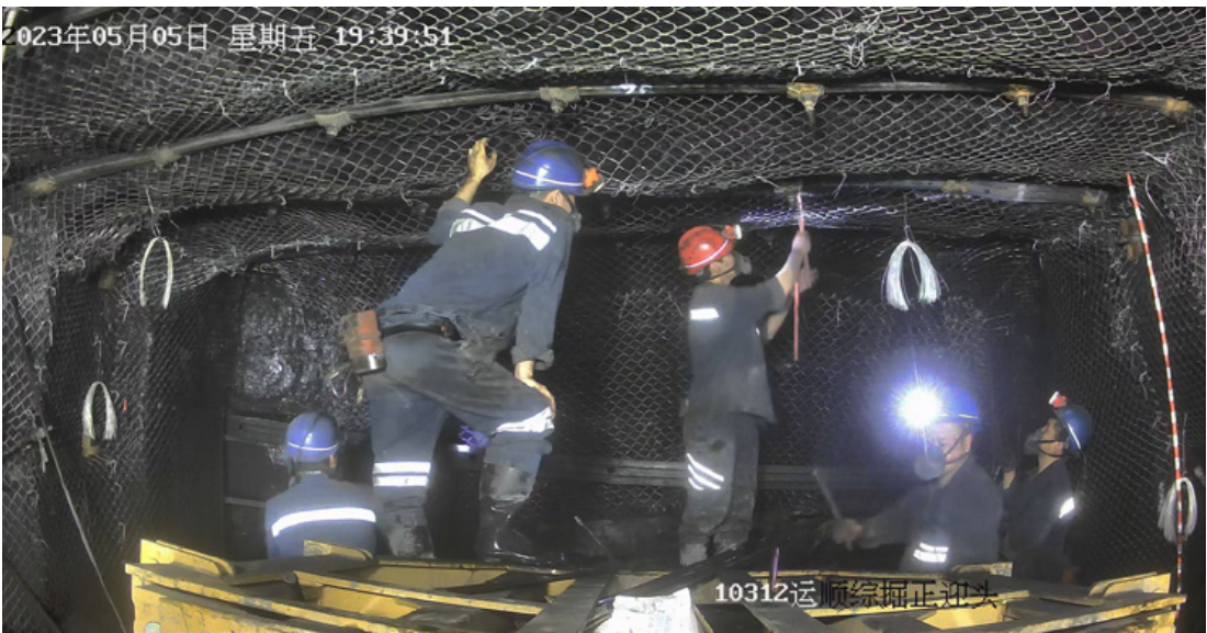
图 6-7 掘进作业施工现场
