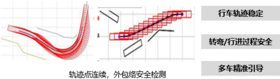
图 11-5 基于车辆运动学的全局路径设计
